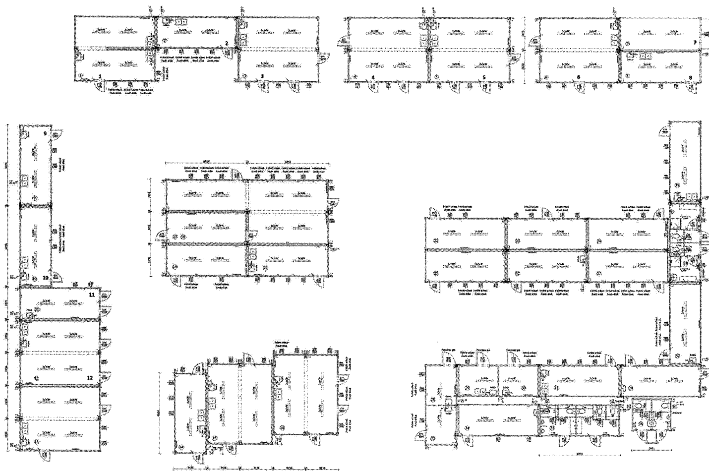
Teleki téri ideiglenes piac konténer elhelyezési terv
