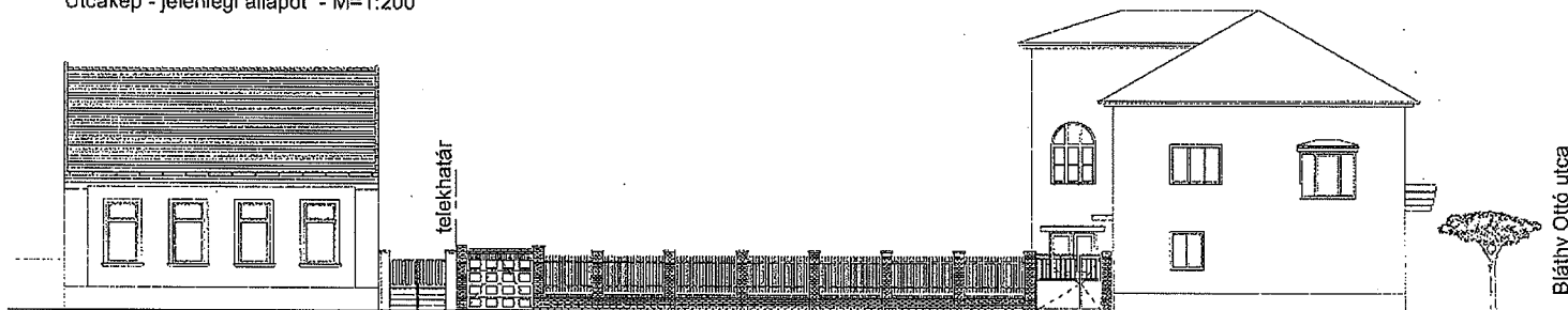
Utcakép - jelenlegi állapot - M=1:200
