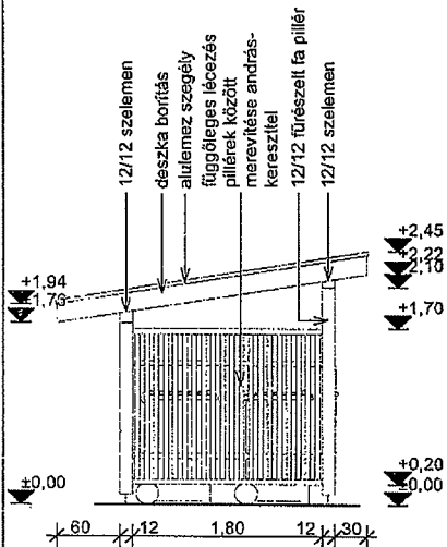
DÉLNYUGATI HOMLOKZAT M=1:50
