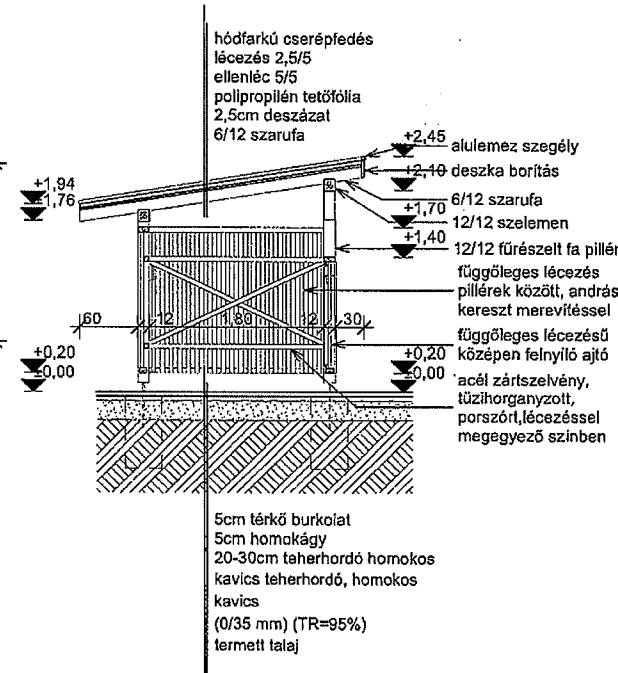
DÉLKELETI HOMLOKZAT M=1:50
