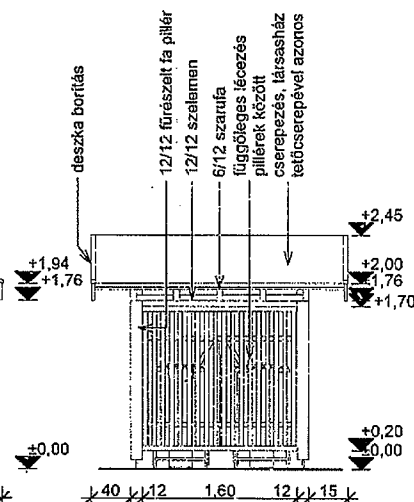
ÉSZAKNYUGATI HOMLOKZAT M=1:50
