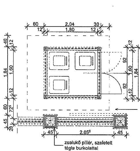
ALAPRAJZ M=1:50
