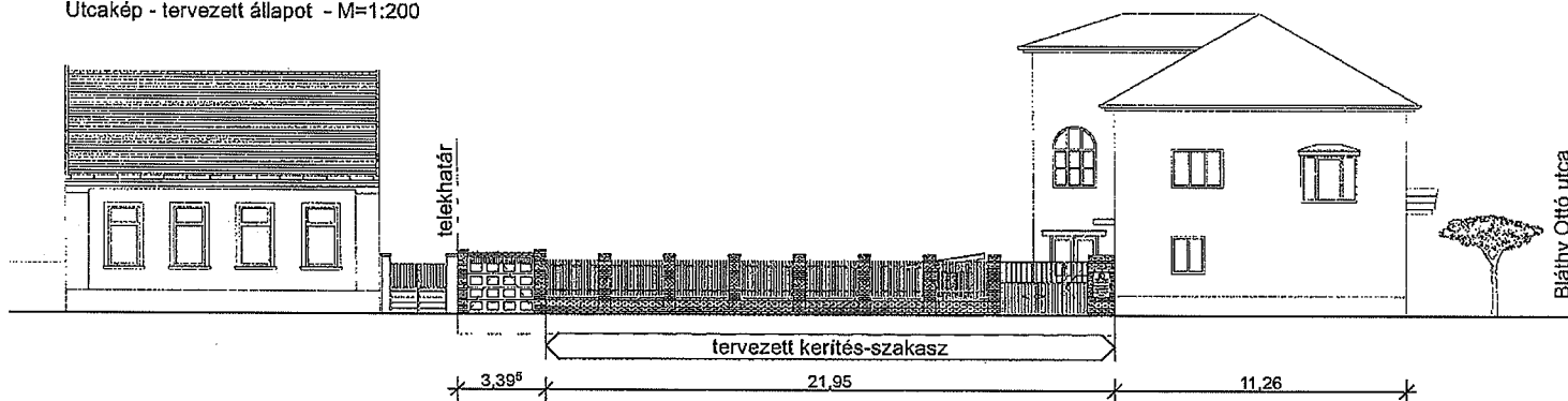
Utcakép - tervezett állapot - M=1:200
