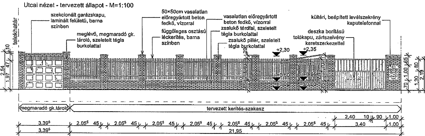
Utcai nézet - tervezett állapot - M=1:100
