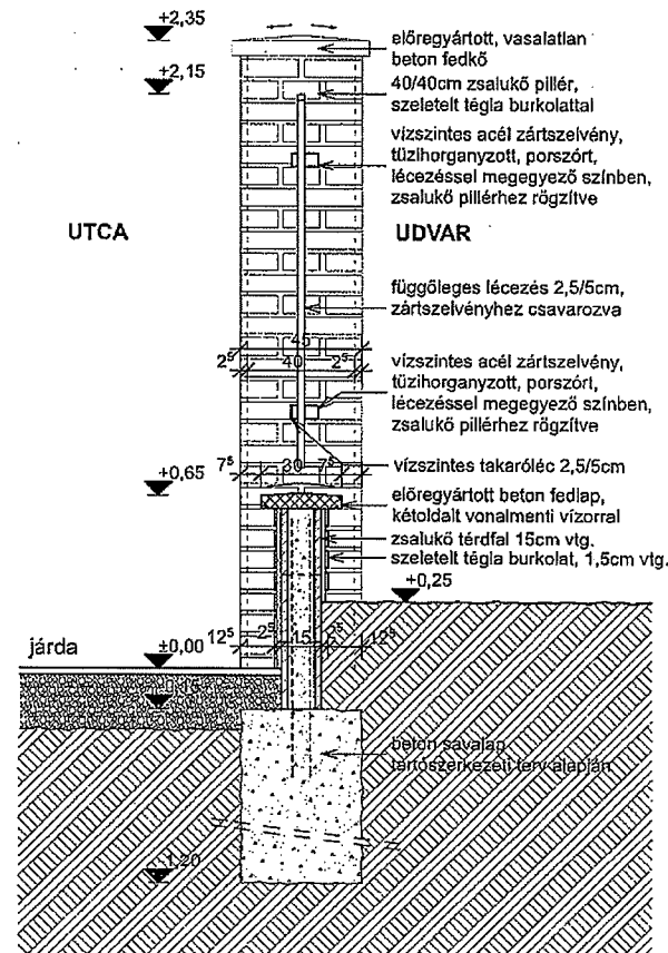
Kerítés metszet - tervezett állapot - M=1:20
