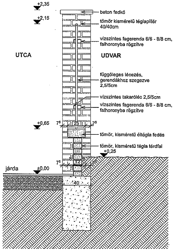
Kerítés metszet - jelenlegi állapot - M=1:20
