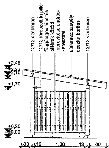
ÉSZAKKELETI HOMLOKZAT M=1:50
