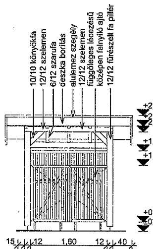
DÉLKELETI HOMLOKZAT M=1:50
