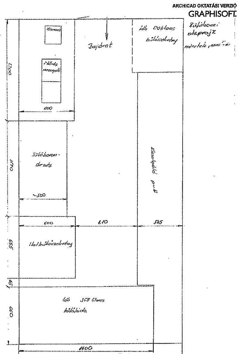
Alaprajzi elrendezés
