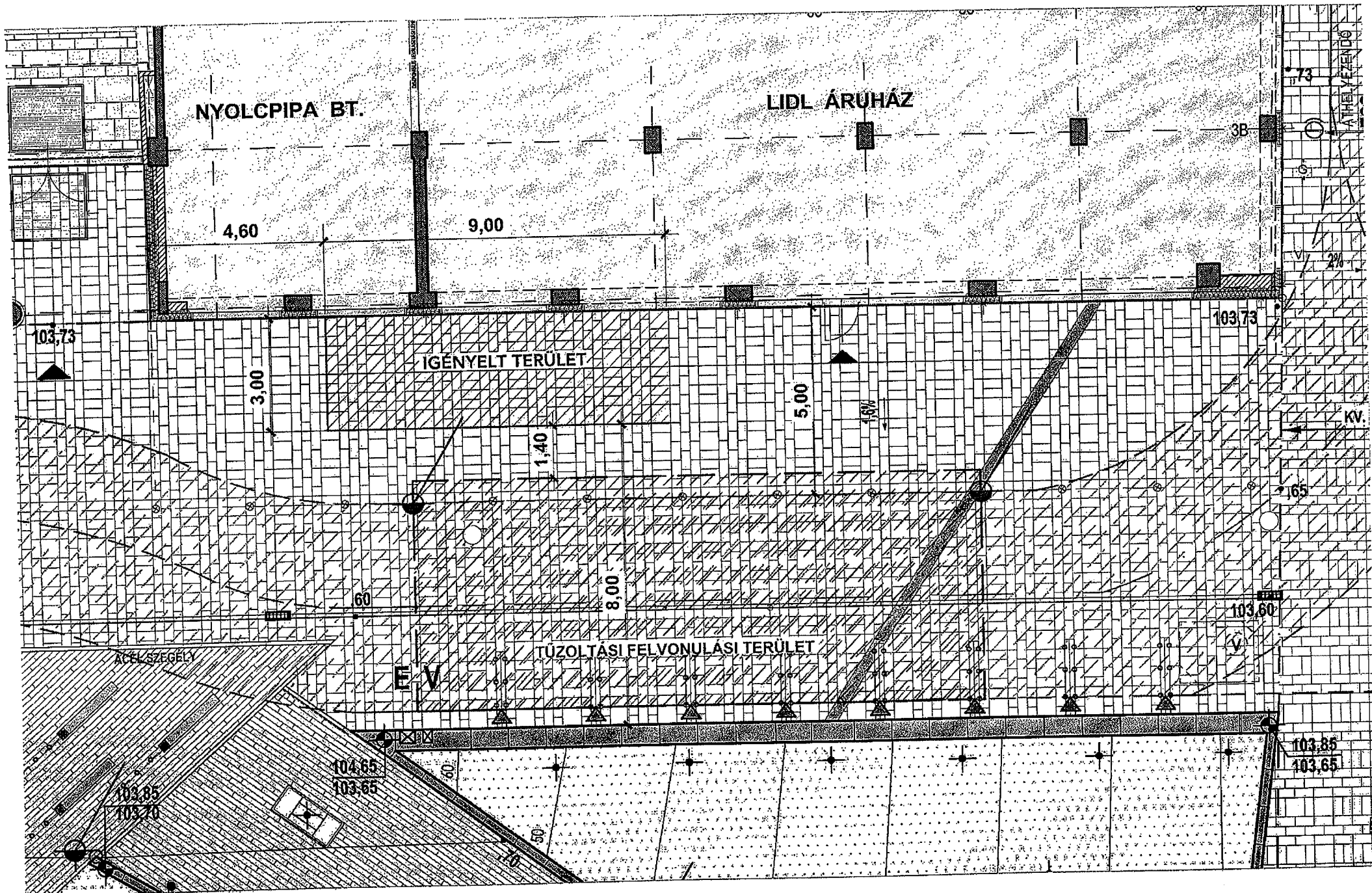
NYOLCPIPA BT. TERASZ KÉRELEM ALAPRAJZA M=1:125
