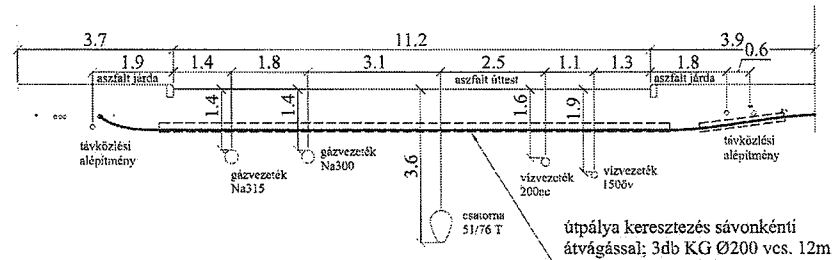
Bp. VIII. Diószegi utca keresztezés M1:100
