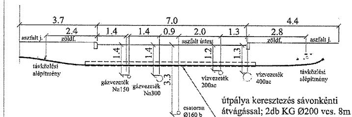
Bp. VIII. Delej utca keresztezés M1:100
