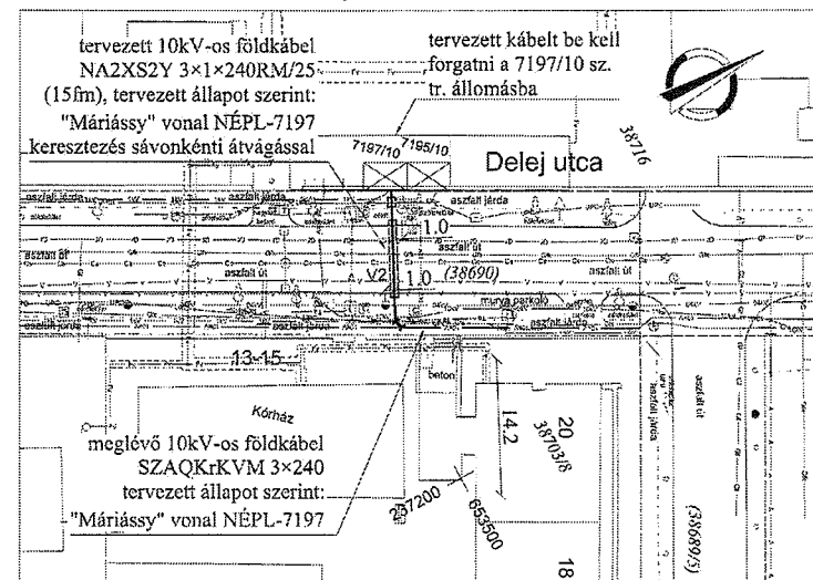
Egyesített közműves nyomvonalrajz, csak az érintett közművek nyomvonalait tartalmazza! M1:500
