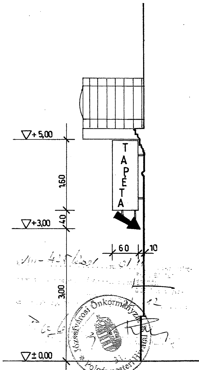
metszet M=1:50
