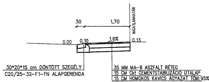
KAPUBEHAJTÓ II. HOSSZ-METSZET A TENGELYVONALBAN
