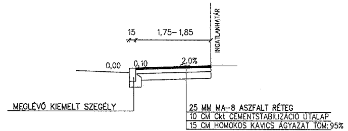
JÁRDA HOSSZ-METSZET
