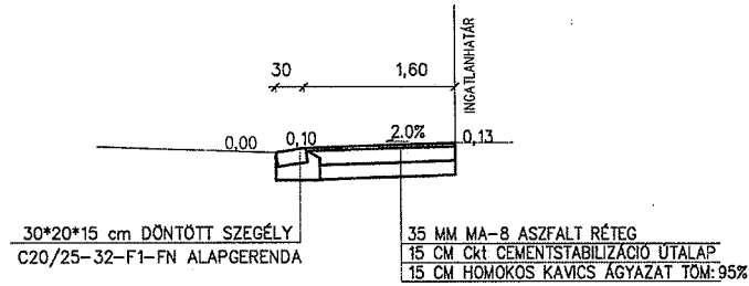
KAPUBEHAJTÓ II. HOSSZ-METSZET A TENGELYVONALBAN
