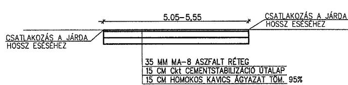
KAPUBEHAJTÓK KERESZT-METSZET
