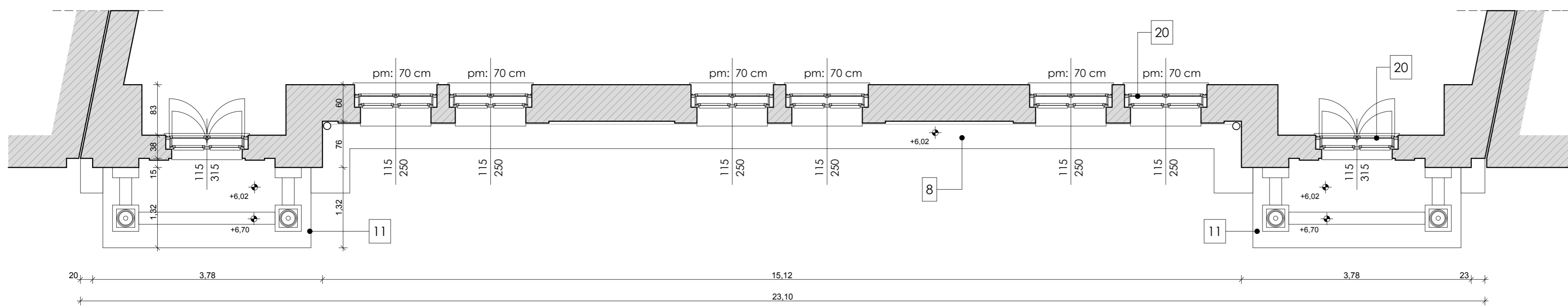
A - A vízszintes metszet
