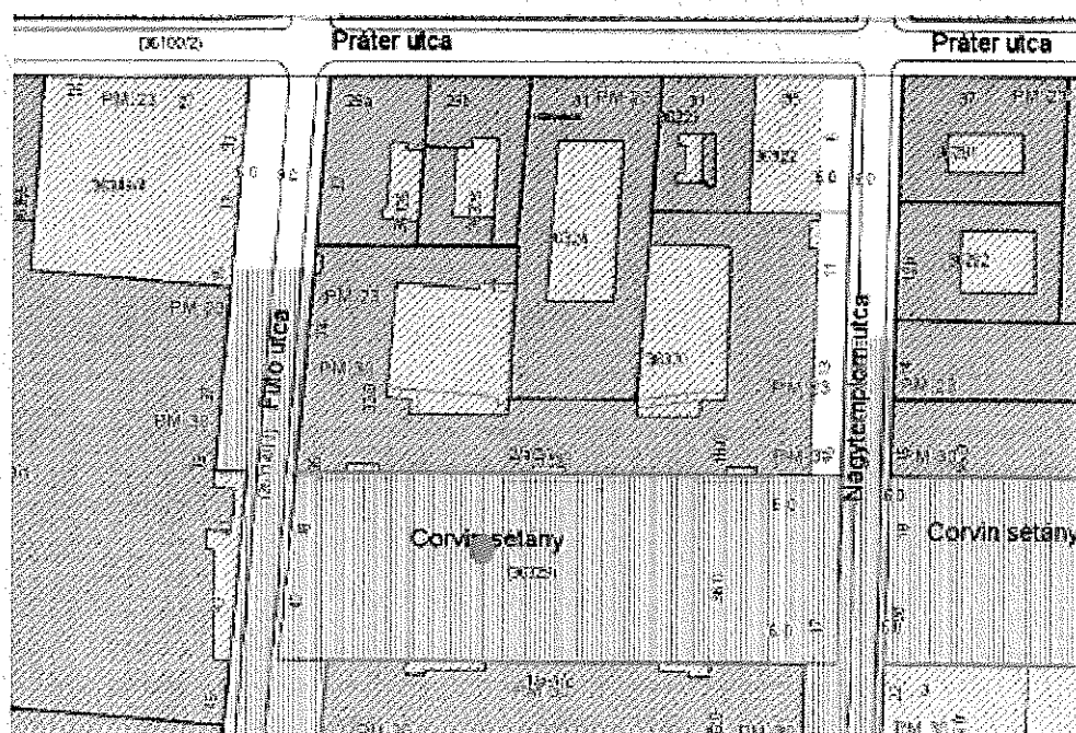
119-es számú „CorvinPláza” kamerahelyszín alépitmény szakasz és betáplálási pont
