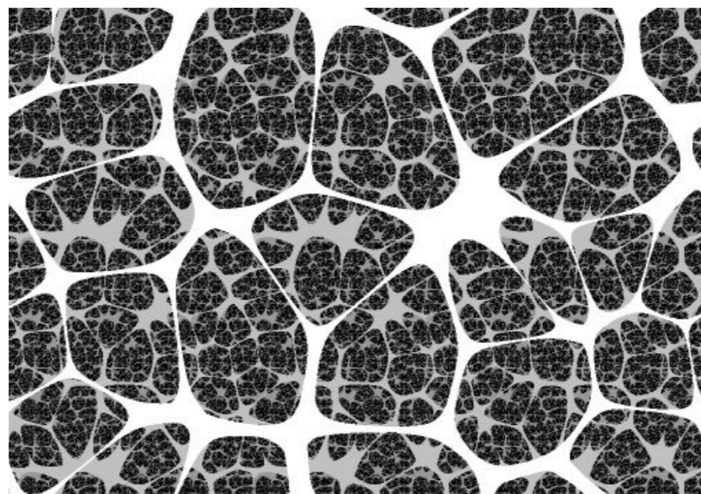
FRAKTÁLGEOMETRIA
