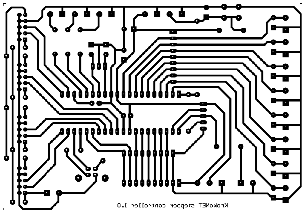
NYOMTATOTT ÁRAMKÖR
