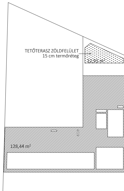
TETŐTÉR 1 (6. EMELET)
