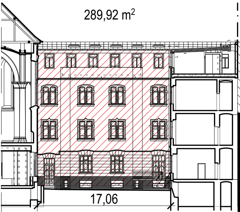
Lift udvar Keleti homlokzat
