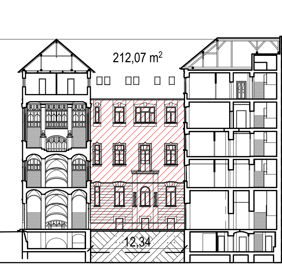
Szent Ignác Kollégium udvar Nyugati homlokzat
