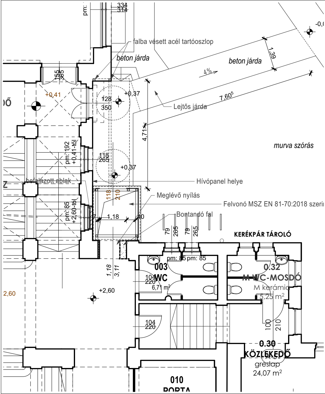
Földszinti alaprajz
