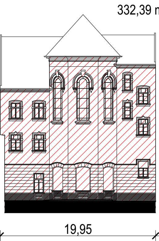
Mária utcai homlokzat
