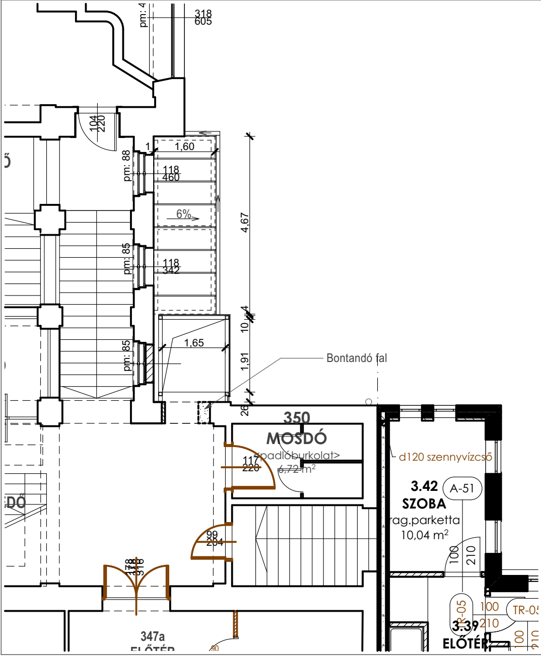
3. szinti alaprajz
