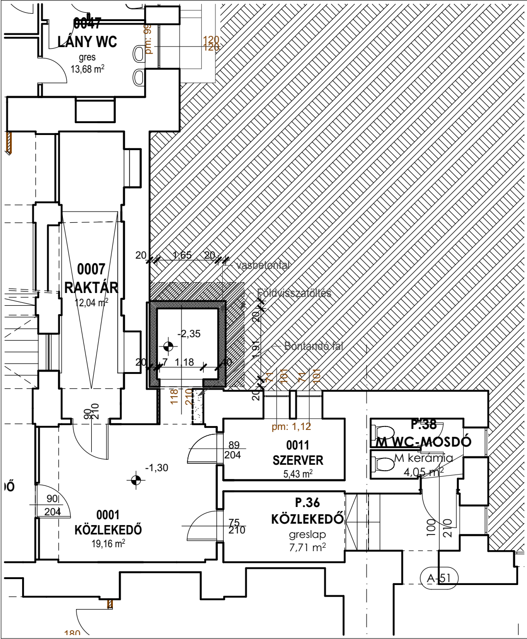
Alagsor alaprajz
