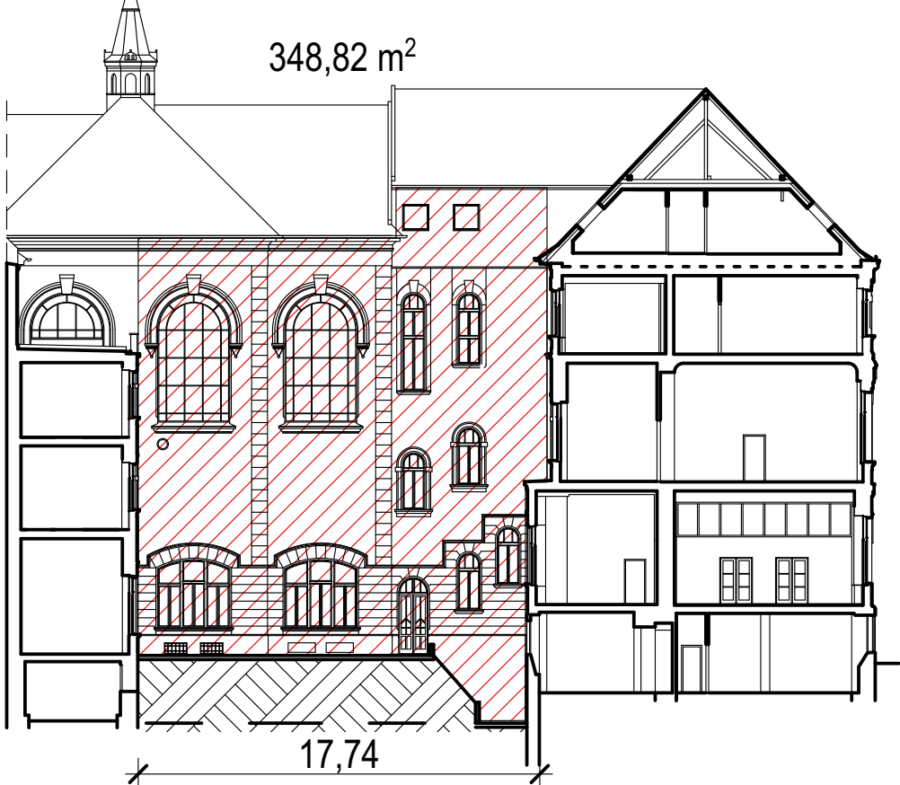
Szent Ignác Kollégium udvar Déli homlokzat
