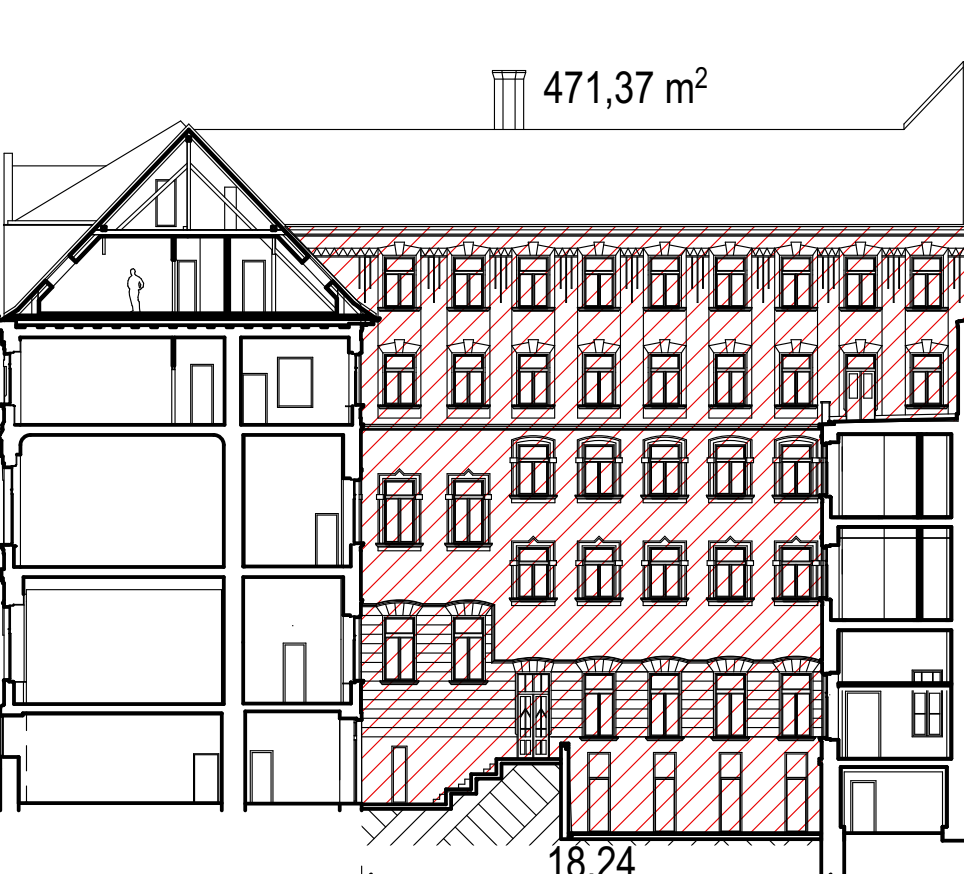
Szent Ignác Kollégium udvar Északi homlokzat
