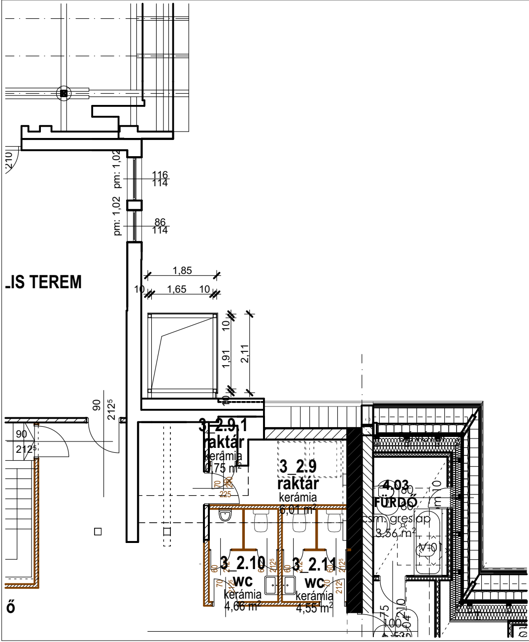
4. szinti alaprajz
