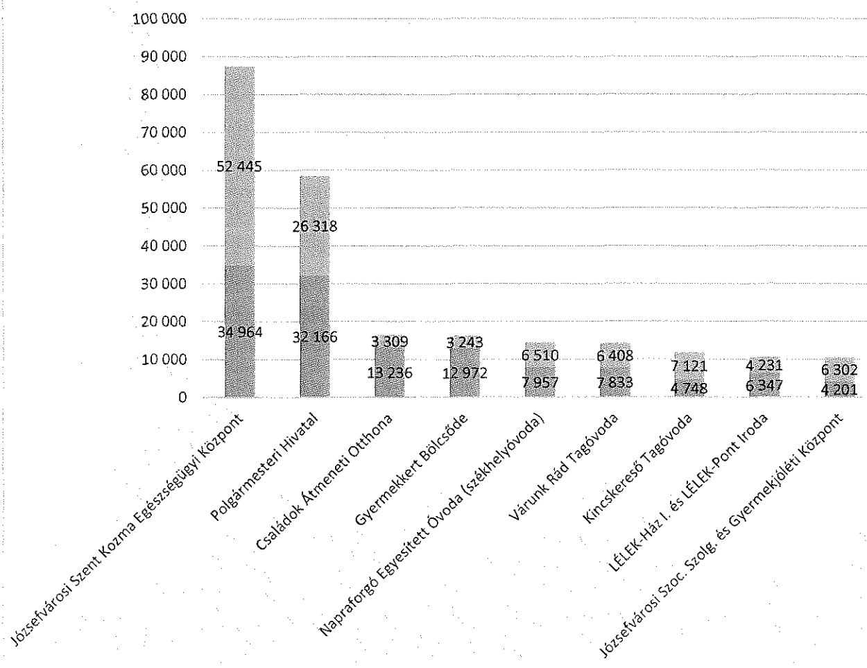
18. ábra: Energiahatékonysági beruházásokkal elérhető megtakarítások a gázfogyasztásban Jelenlegi fogyasztás: teljes oszlopmagasság; Elérhető megtakarítás: sárga oszlop; Beruházások utáni fogyasztás: kék oszlop
