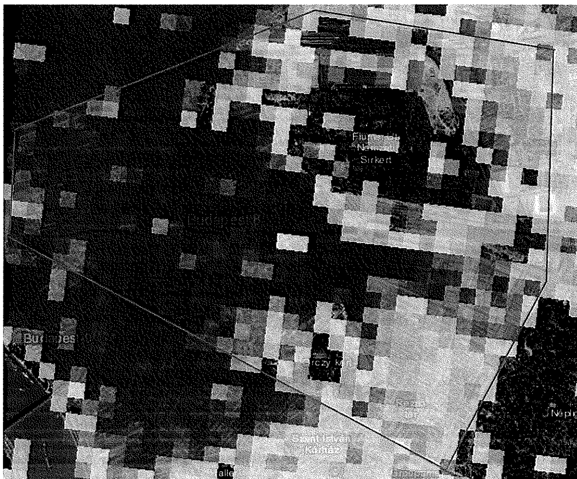
1. ábra: Az VIII. kerület épületeinek hőigény-sűrűsége ( \text{m}^3/\text{ha} ) - a sötétebb árnyalatok nagyobb sűrűséget jelölnek (HOTMAPS szoftver)
