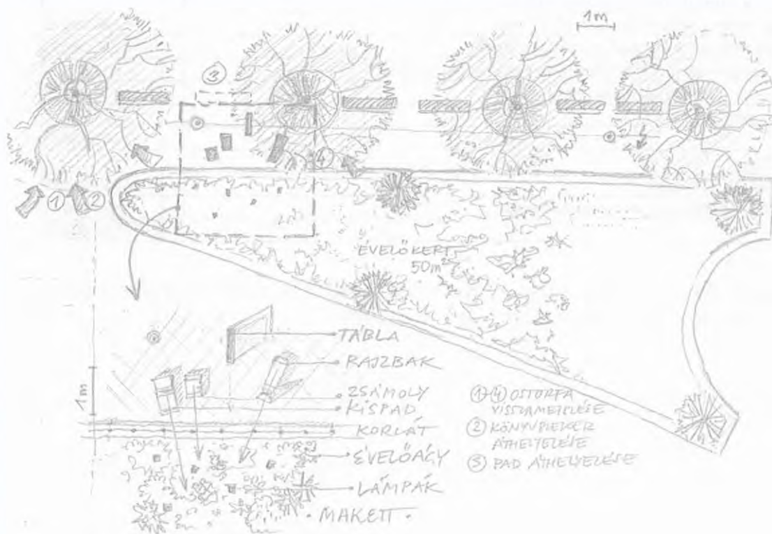
Helyszínrajz a modell (makett kiemelésével)
