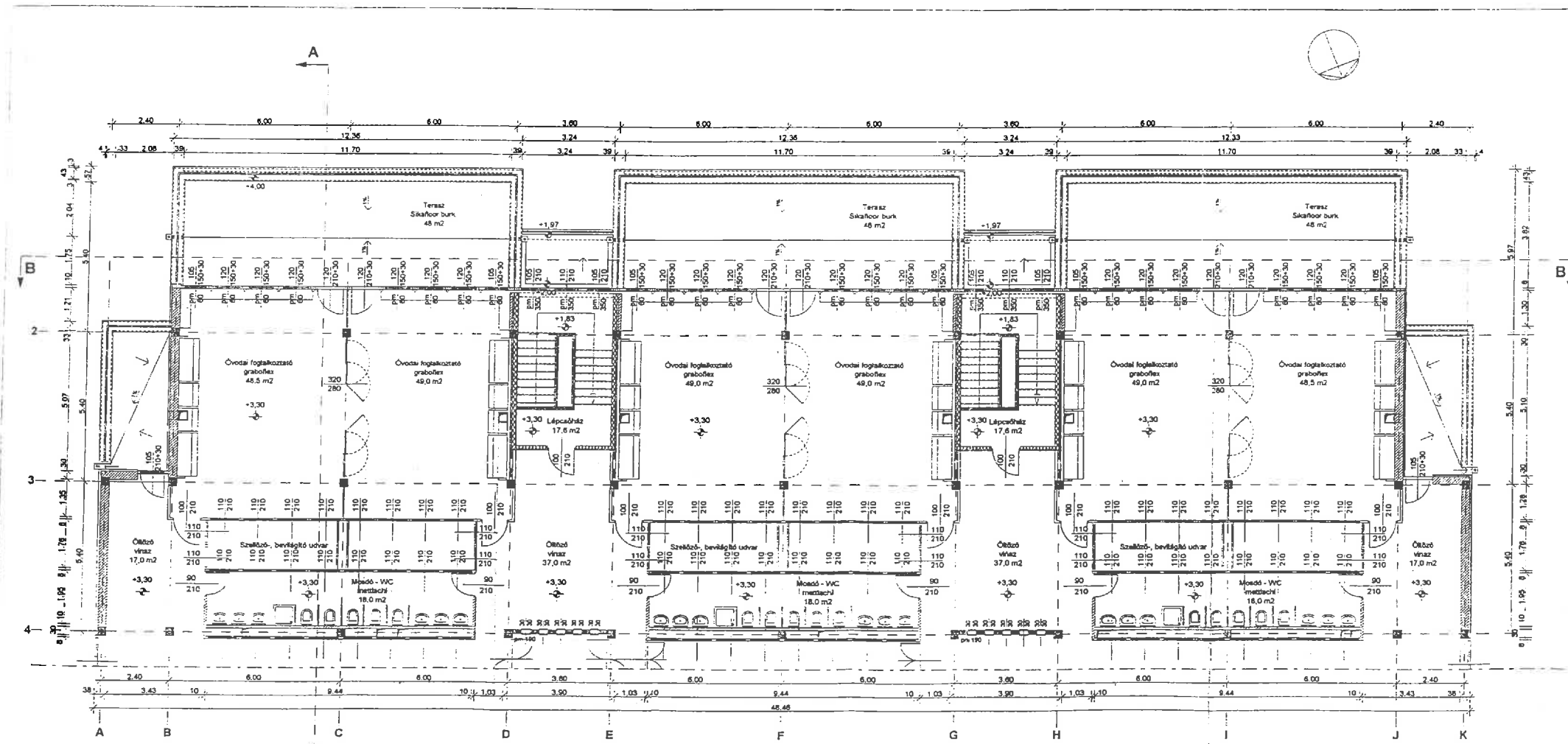
Meglévő emeleti alaprajz M 1:100
