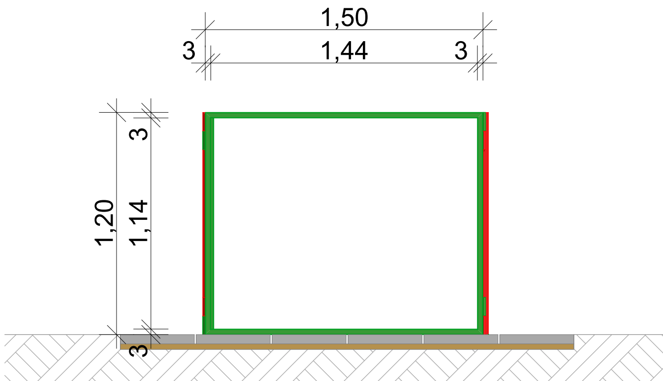
ELÖLNÉZET
