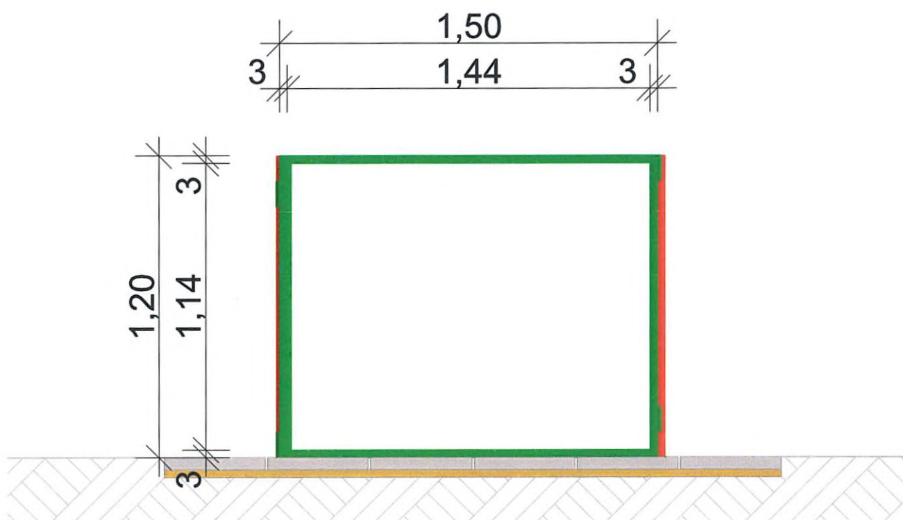
ELÖLNÉZET
