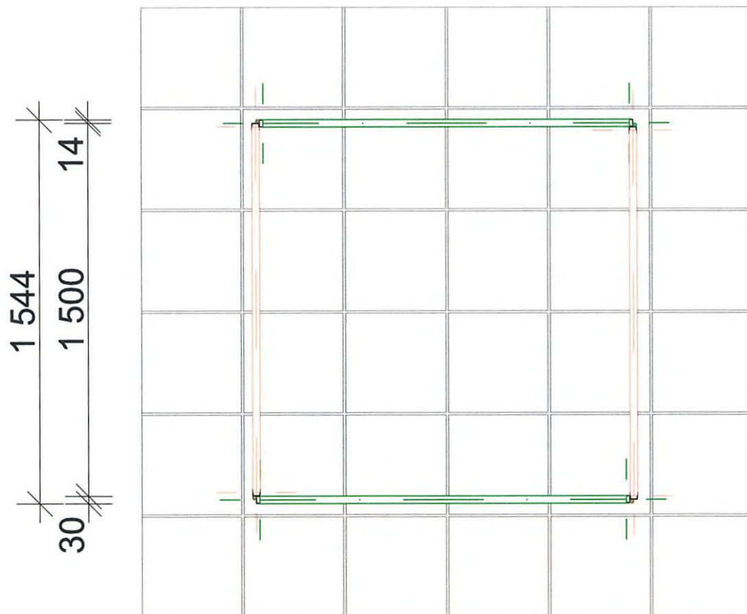
FELÜLNÉZET
