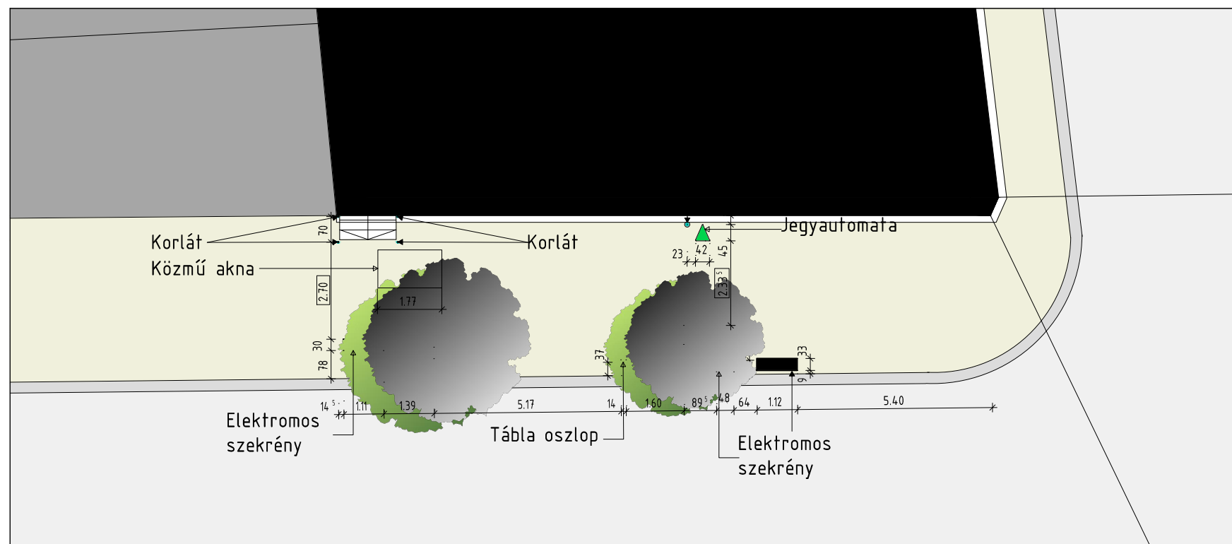
Részletes helyszínrajz
